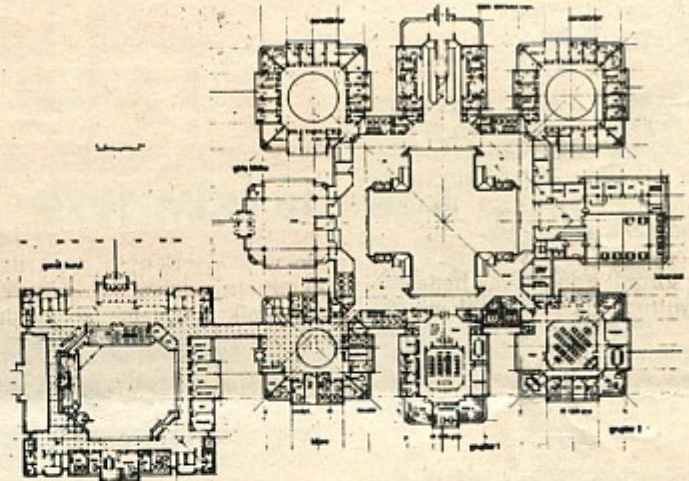
1. Ödül - Zemin Kat Planı
